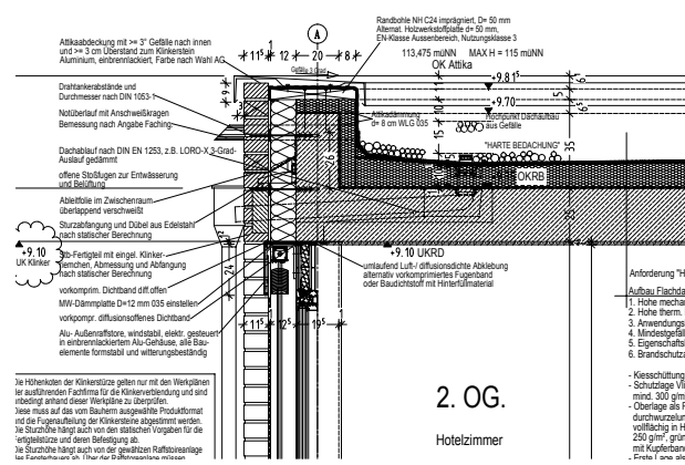
Fassadenausschnitt A1 M 1:10
