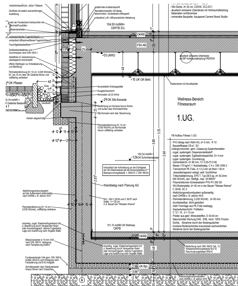
Fassadenausschnitt A1 M 1:10
