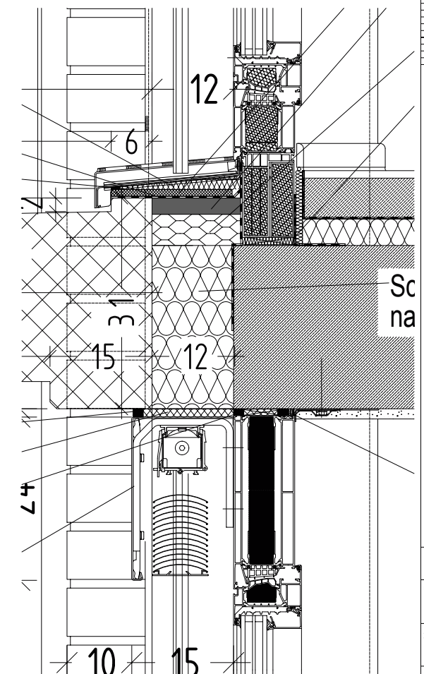
Fassadenausschnitt A1 M 1:2
